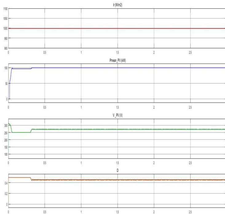
Fig 13- Solar PV output Parameters
